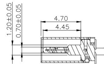
剖视“A-A” 比例 1:1
